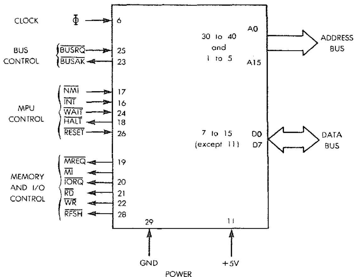
Fig. 2.33: Z80 MPU Pinout
