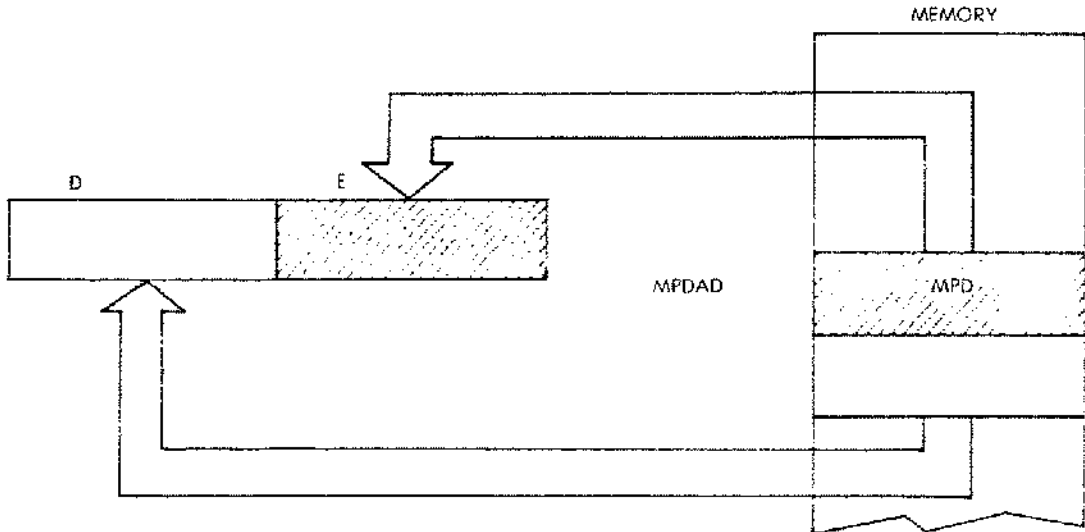
Fig. 3.16: LD DE, (MPDAD)
