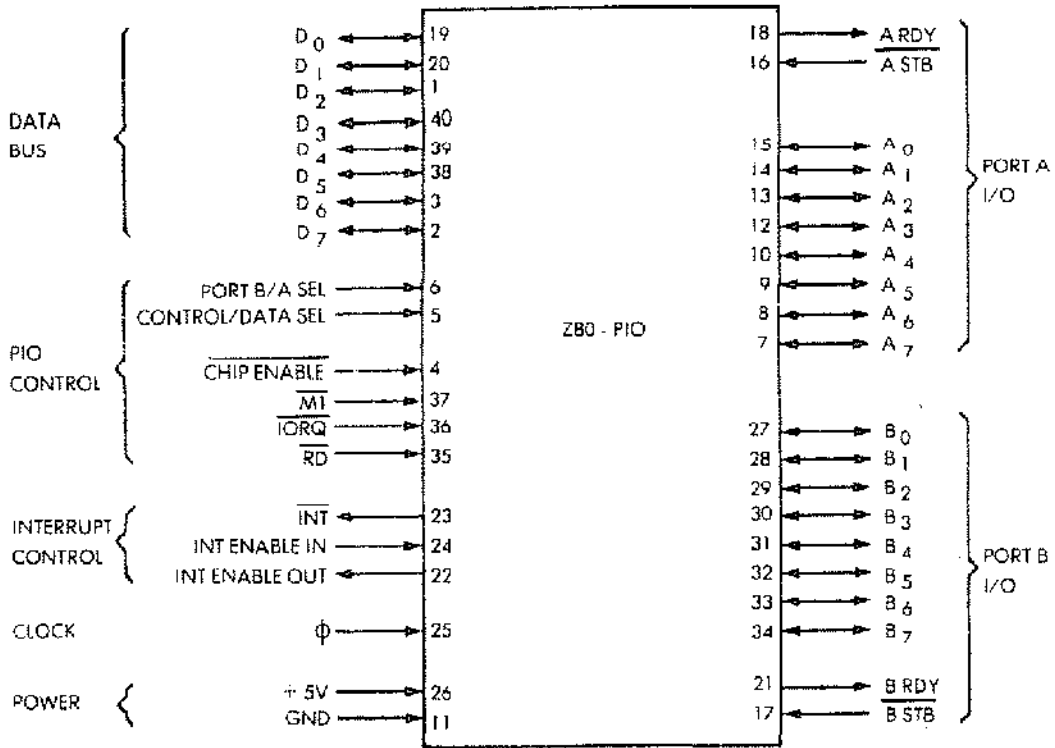
Fig. 7.6: Z80 PIO pinout
