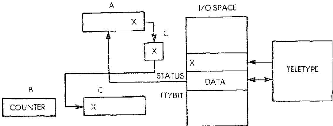
Fig. 6.15: Teletype Input
