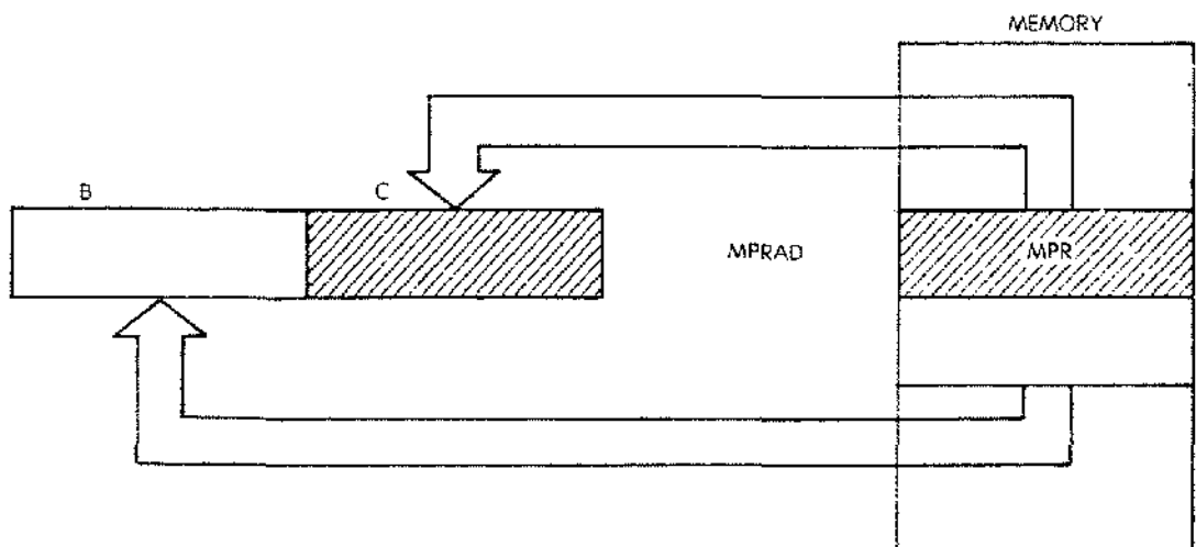
Fig. 3.15: LD BC, (MPRAD)
