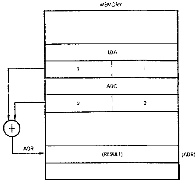
Fig. 3.10: Storing BCD Digits
