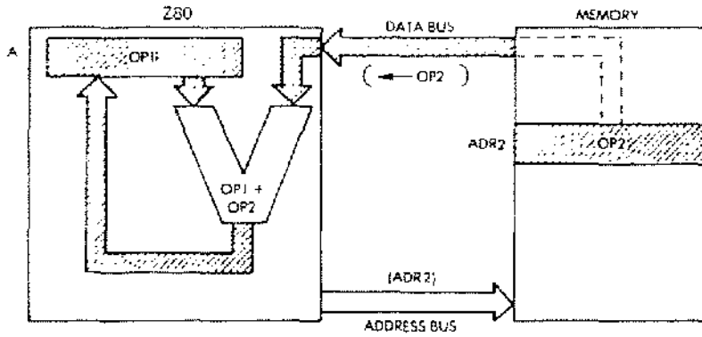
Fig. 3.3: ADD A, (HL)
