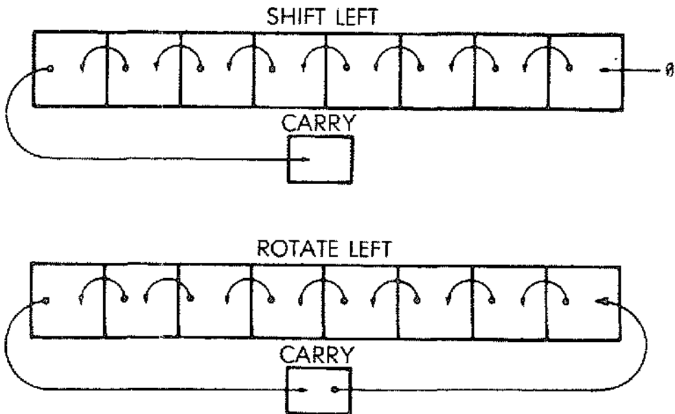
Fig. 3.17: Shift and Rotate
